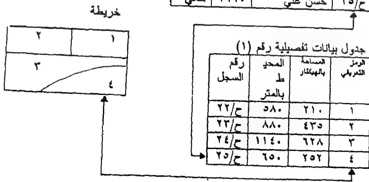
شكل (١٣): يوضح نموذج تخطيطي لتصميم انترابطي في قواعد المعلومات
