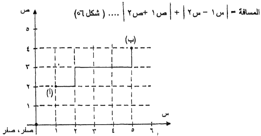
شكل (56): طريقة مانتن المتريية لحساب المسافة بين النقط
