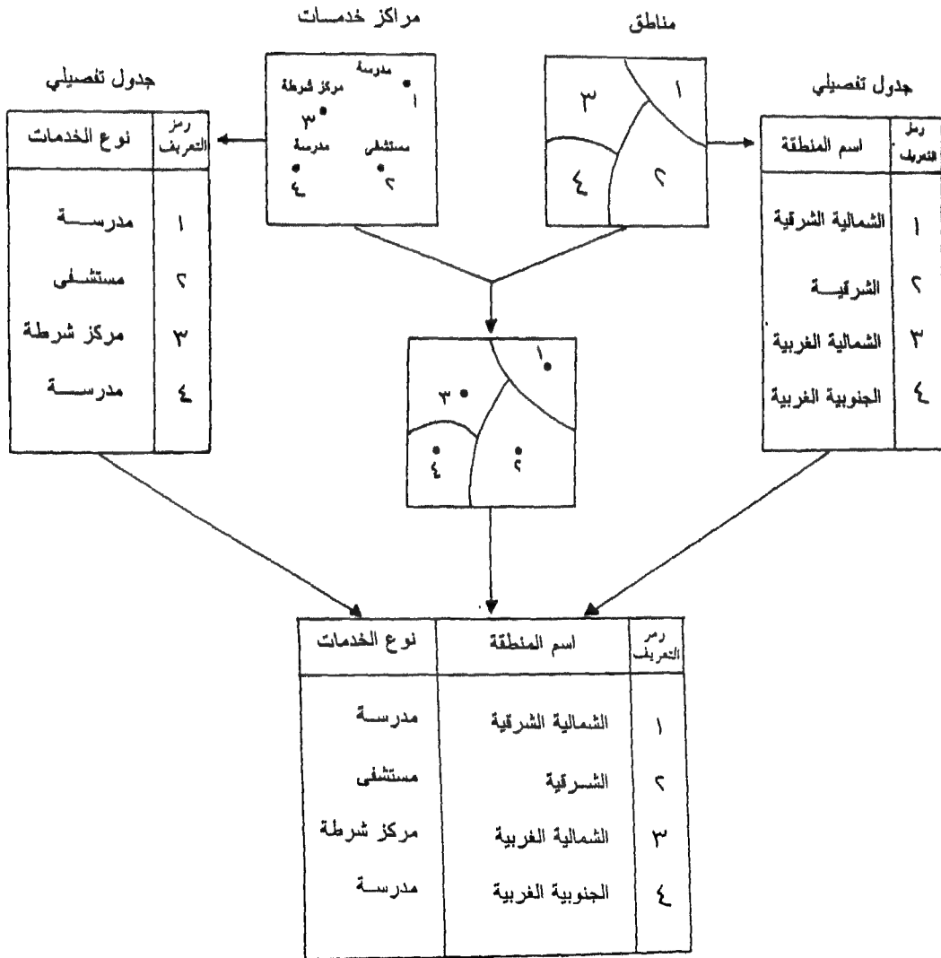
شكل (٦): عملية مطابقة البيانات الطوبولوجية من طبقتين معلومتين مختلفتين ( عناصر نقطية مع مساحة)
