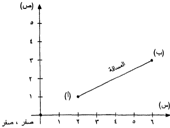
شكل (55): طريقة فيثاغورث لحساب المسافات بين النقاط
