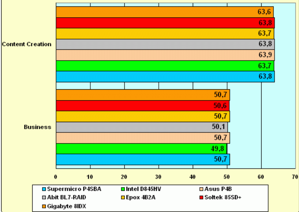
Ziff-Davis Winstone 2001
